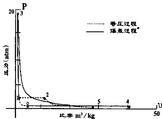
图 5 等压和爆轰热力循环比较
