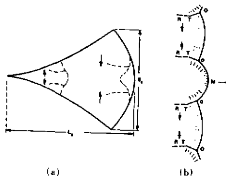
图 3 Schematic of instantaneous profile of a multi-dimensional detonation front and detonation cell etched on a deposit on tube wall: OT — transverse shock; TR — trailing acoustic waves; OM — Mach stem; O — triple point; ... — reaction zone; ||| — unreacted gas mixture [8] . 换, 则爆轰波可以看作一个固定间断面。可燃气体以速度 u_1 进入间断面, 燃烧产物以速度 u_2 离开; 气体由状态 1 变成状态 2。图 4 表示了爆轰波的分析模型, 控制体和状态参数。包含爆轰波作控制体则可得质量、动量和能量守恒方程。
