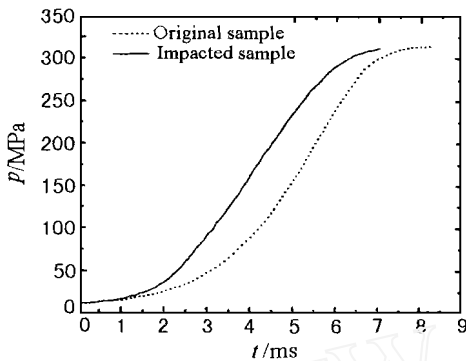
图 5(a) p-t 曲线
