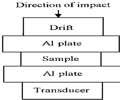
图1 撞击试验简图
