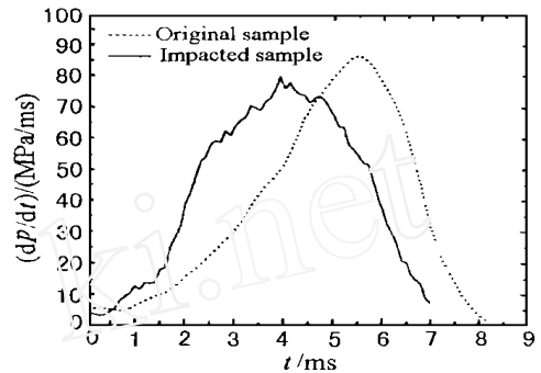
图 5(b) (dp/dt)-t 曲线
