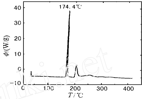
图 4(b) DSC 曲线 Fig. 4(b) DSC curve
