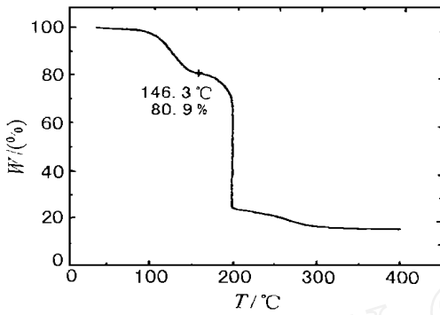
图 4(a) TG 曲线 Fig. 4(a) TG curve
