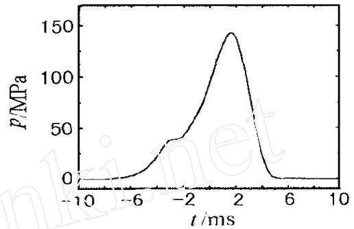
图2 加载曲线
