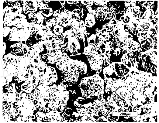
图 3(b) 损伤试样微结构形貌
