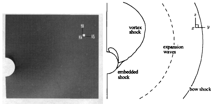
图 12 x/D = 5.5 剖面处的密度云图 (情况 3)
