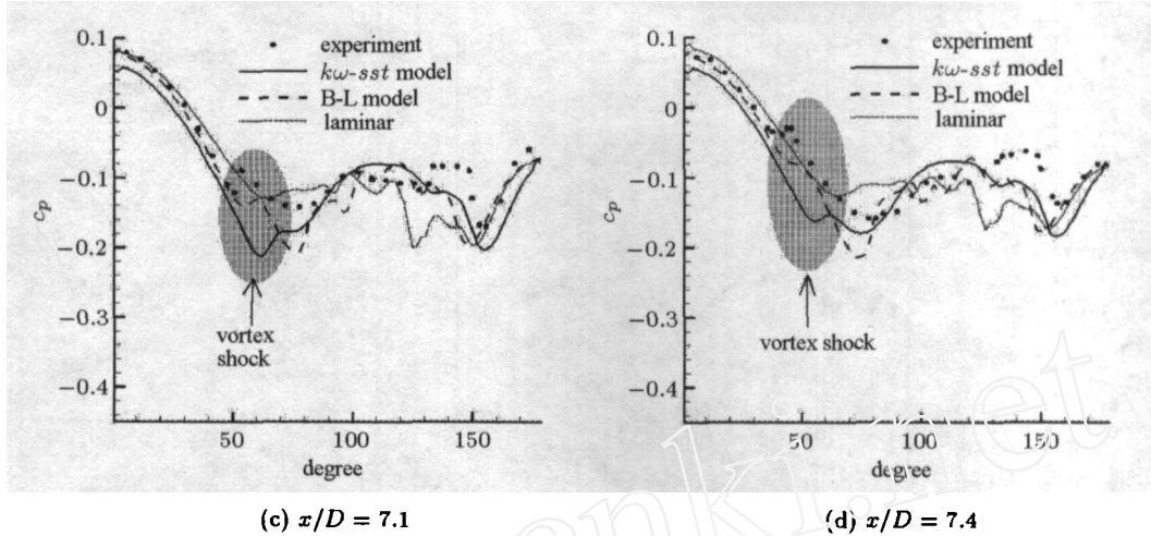
图 14 环向表面压力分布 (情况 4)
