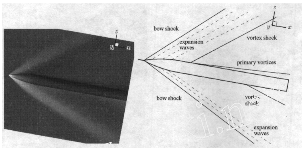
图 5 纵剖面密度云图 (情况 1)
