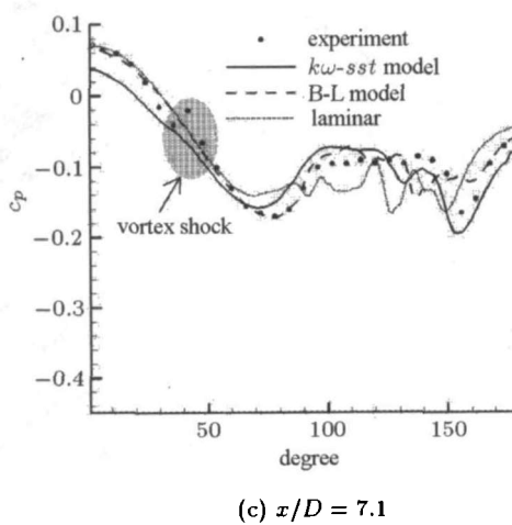
图 9 环向表面压力分布 (情况 2)
