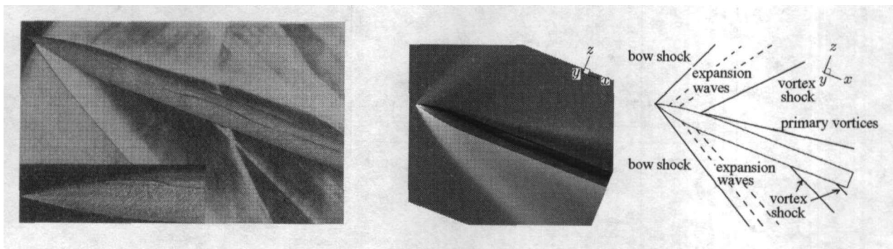
(a) 条纹照相与油状流动合成图 (情况 5)
