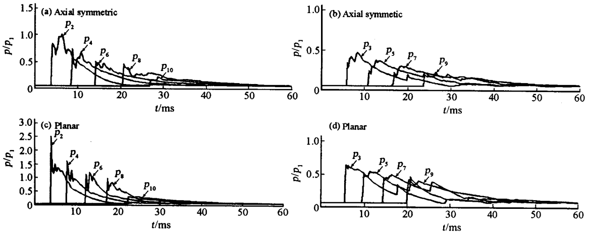
图 10 压力-时间曲线 ( D/d=2, L/d=2 )
