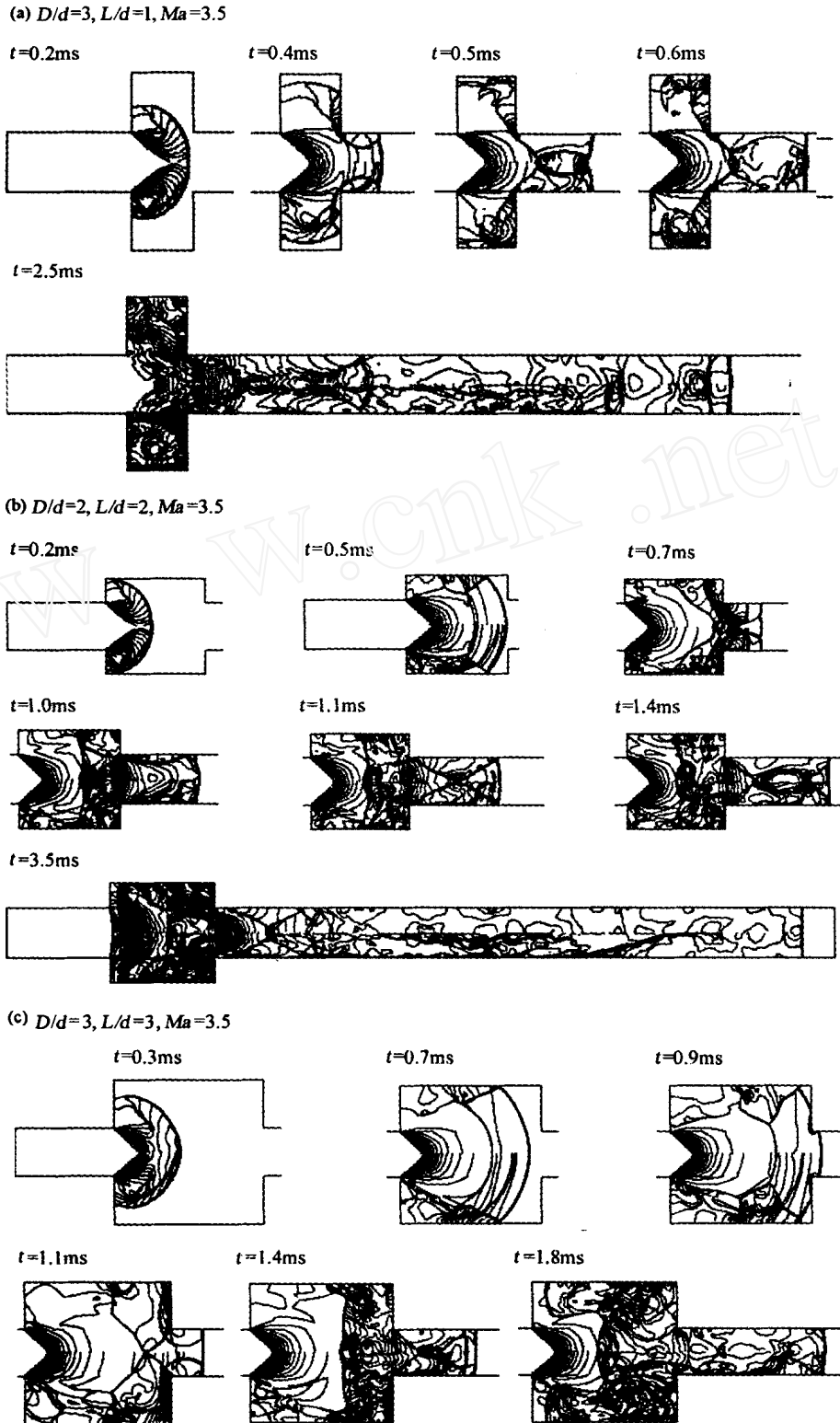
图 6 压力分布(上半)和密度分布(下半)
