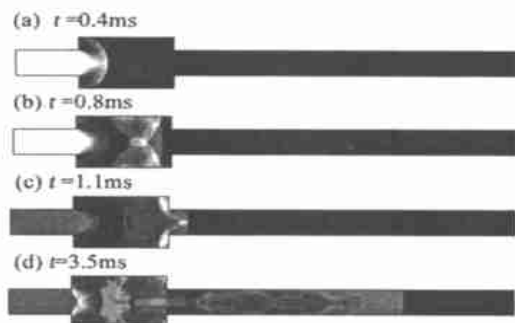
图 1 激波 ( Ma = 3.0 ) 在扩容室内传播不同时刻的密度分布 Fig. 1 Sequential distribution of density contour
