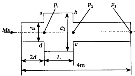
图4 扩容室结构和特征尺寸
