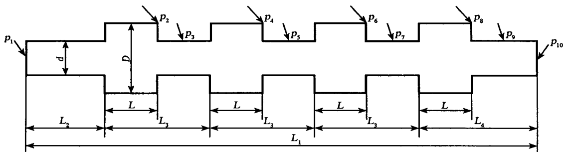
图 9 四级扩容室串联结构示意图
