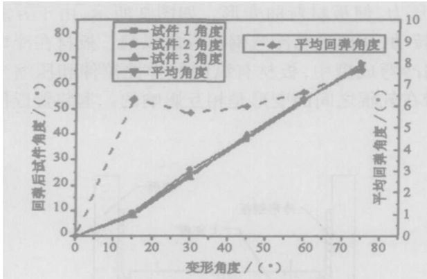
图5 6 mm 钢板试件回弹角度
