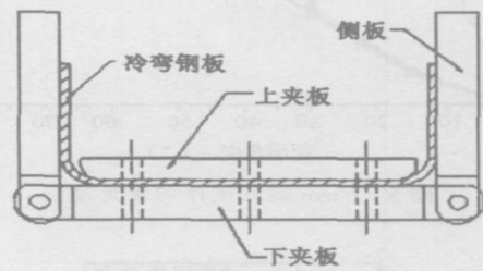
图2 板带装置的变形图
