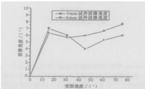
图7 测试试件回弹对比图
