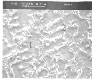
图 8 焊缝组织扫描电镜图
