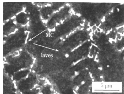
图 10 焊缝区域扫描电镜图——Laves 相
