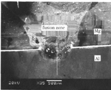
图3 镁铝 TIG-激光复合焊接接头微结构扫描电镜图片 (中间层为铈金属)
