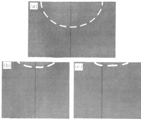
图 7 熔池轮廓实验与数值模拟对比 (白色虚线表示实验测量焊缝轮廓线)
