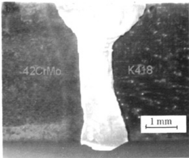
图 5 42CrMo 与 K418 焊缝形貌
