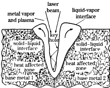
图 1 异种金属激光深熔焊接熔池示意图
