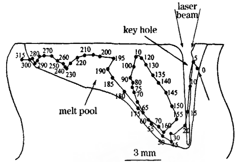
图 6 熔池中钨颗粒的运动轨迹
