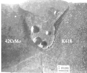
图 9 焊缝根部气孔
