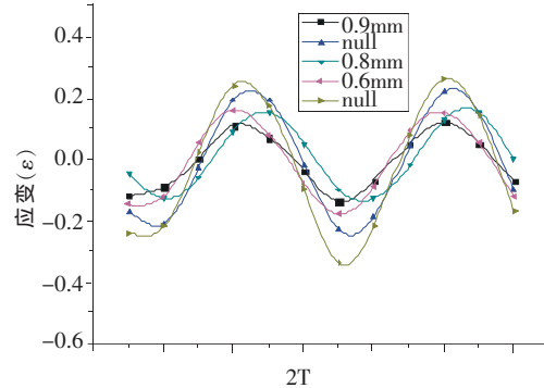
(d) 电阻点焊疲劳试验 961.2 万次采样
