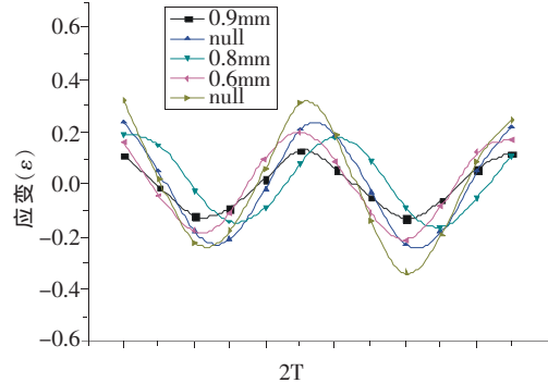
(c) 电阻点焊疲劳试验 64 万次采样
