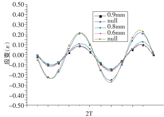
(a) 氩弧点焊疲劳试验 64 万次时采样
