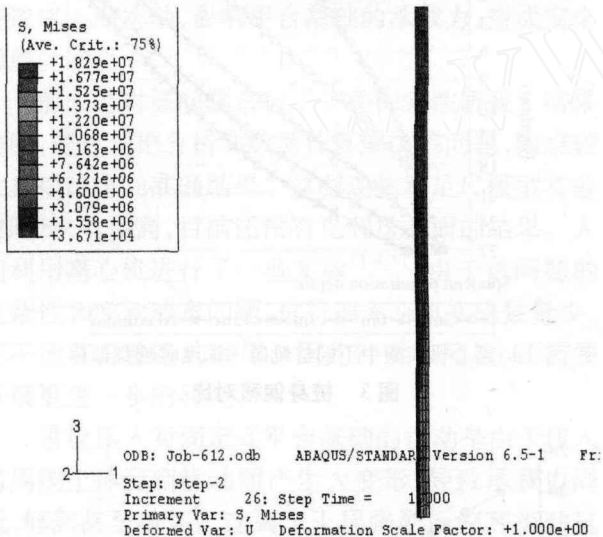
图6 桩基应力场
