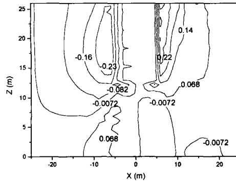
图7 y=0 平面土体水平位移场
