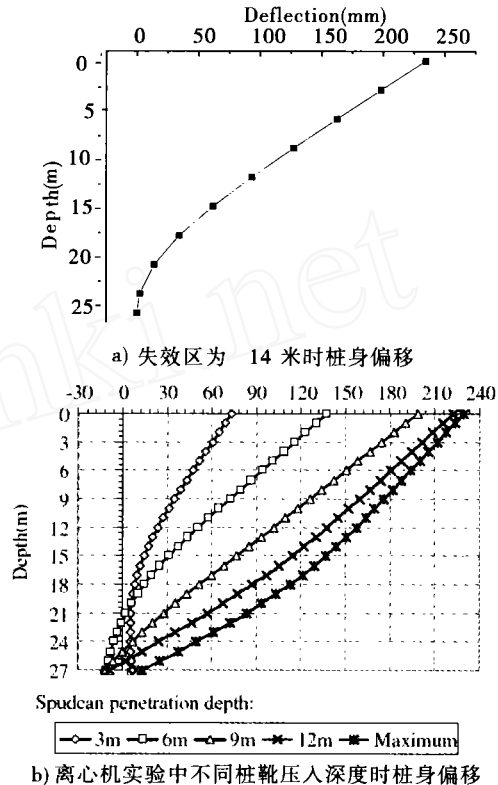
图 3 桩身偏移对比
