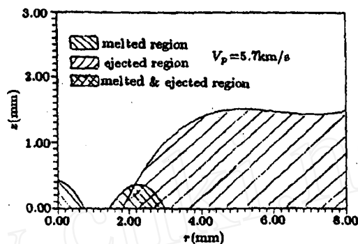
图 6(b) 熔化区与反向飞溅区
