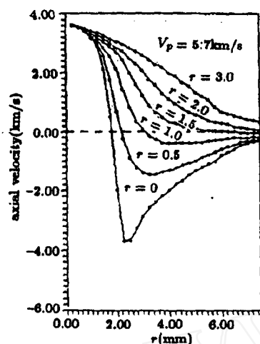
图 6(a) 不同 z 剖面质点轴向速度 沿径向分布
