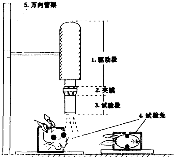
图 3 BST- II 型结构示意图
