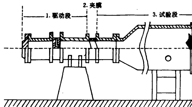
图 2A BST- I 型结构示意图
