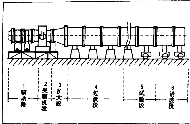
图 1 BST-I 型结构示意图
