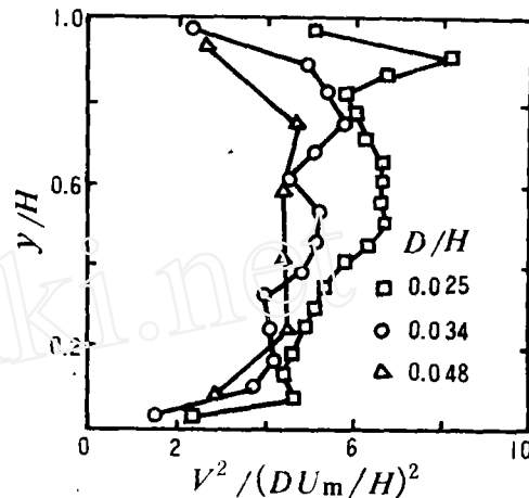
图1 无粘颗粒流脉动速度均方值的分布
