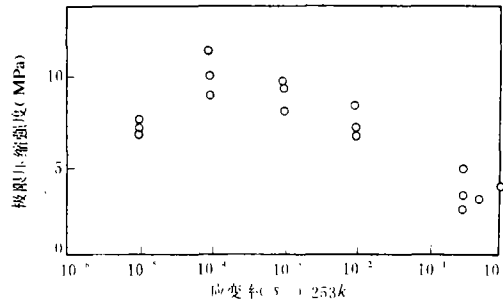
图1 冰的极限压缩强度与应变率的关系
