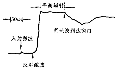
图2 反射段横向窗口的辐射信号(032*)
