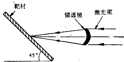
图 2 靶材与光束聚焦位置图
