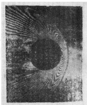
图2 采用平行光穿越实验区的光路(物投影在漫射板上)如图4所示拍摄的流场照片 ( M=2.5 )
