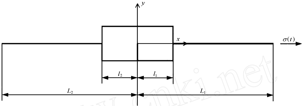
图 4 几何模型
