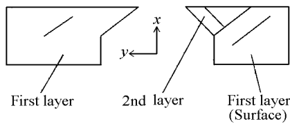
图 14 断开后的 [30_2/-30_2]_s 和 [45_2/-45_2]_s 层合板示意图
