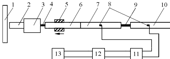
图 1 直拉式 Hopkinson 拉伸杆装置示意图
