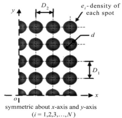
图 1 二维点阵光斑示意图
