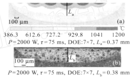
图4 计算所得硬化层形貌(a)与实验所得硬化层形貌(b)
