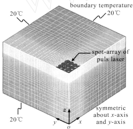
图2 三维有限元模型
