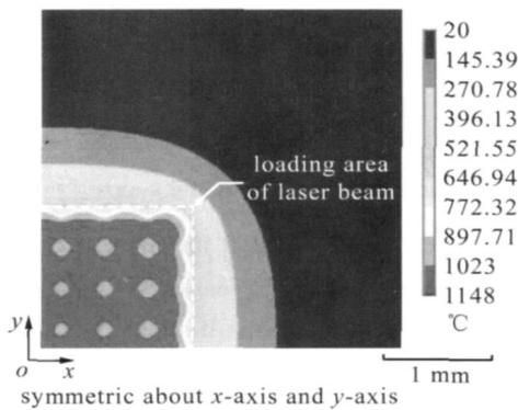
图 7 分布 单脉冲激光作用下的表面温度场
