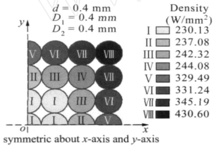
图 6 强度空间分布 示意图
