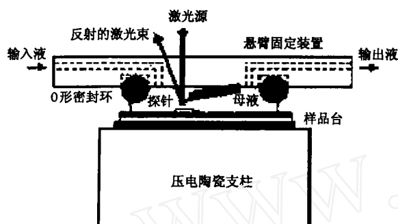
图 1 原子力显微镜研究蛋白质晶体生长工作示意图
