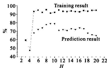
图 1 不同的隐含层单元数 H 对应的训练结果和预测结果
