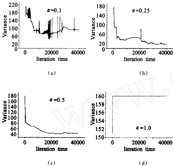
图 2 不同学习步长对应的训练进程
