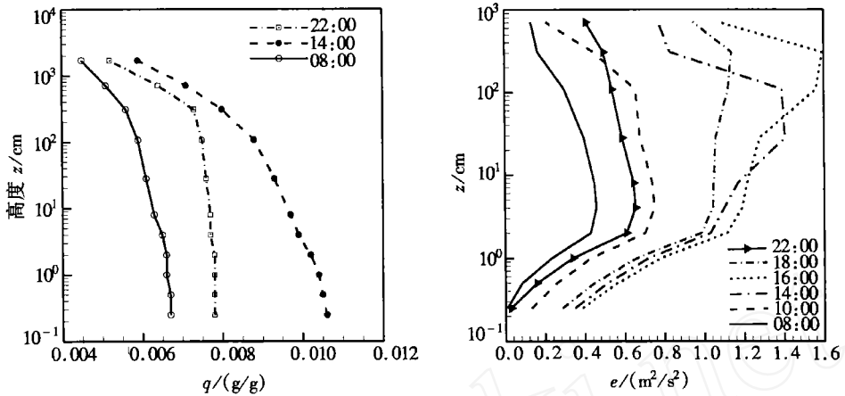
图5 大气比湿模拟值随高度的变化规律 图6 动能 TKE 模拟值随高度的变化规律
