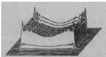
图8 矩形光斑变换系统获得的典型激光功率密度分布
