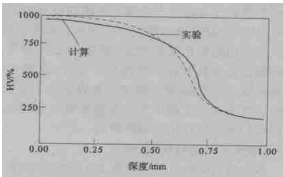
图5 硬度 - 深度计算曲线 (加载值为 50 g)
