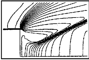
图 10 等压线图(TVD)
