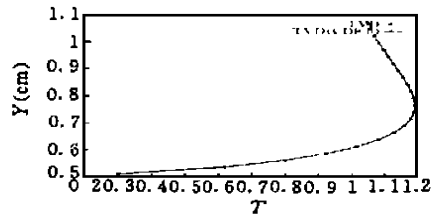
图5 温度分布图
