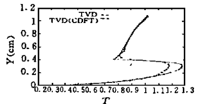
图9 温度分布图
