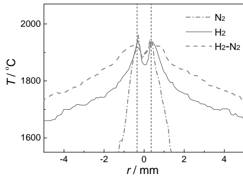
图3 稳定运行条件下再生冷却喷管内壁面温度分布
