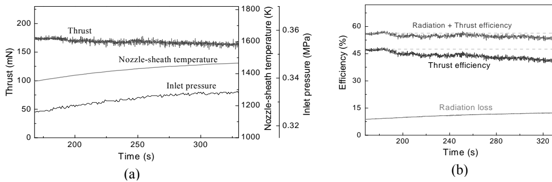
图6 输入电功率 860 W、H 2 /N 2 = 2.8/1.5 slm 条件下，推力器性能及辐射损失变化
