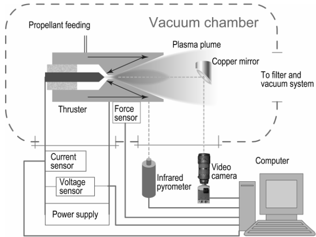
图1 系统示意图
