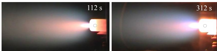
图7 推力器运行中的羽流及喷管照片，运行条件同图6，图中数字表示运行时间
