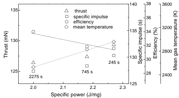
图5 氩推进剂流量100 mg/s、弧电流8 A条件下，推力器性能随运行时间（伏安特性）的变化
