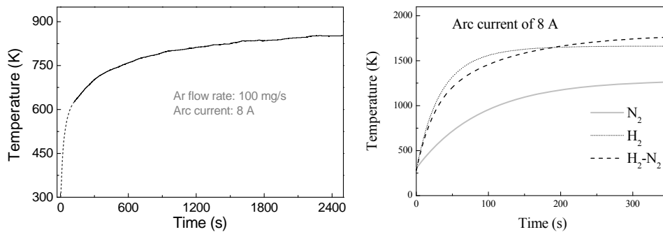
图2 不同推进剂条件下, 再生冷却喷管的温度随点火运行时间的变化。H 2 , 6 mg/s; H 2 -N 2 , 36 mg/s; N 2 , 83 mg/s
