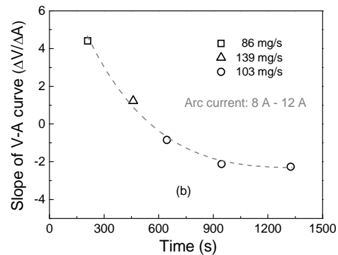
图4 氩推进剂条件下，再生冷却喷管电弧加热推力器伏安特性曲线的斜率随运行时间（喷管温度）的变化
