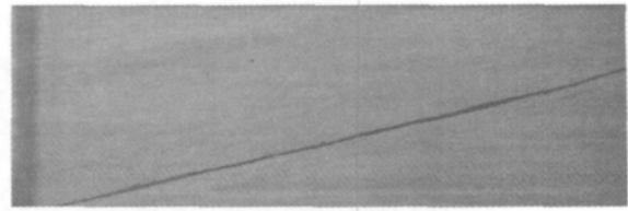
图1 相似材料试验模型图
