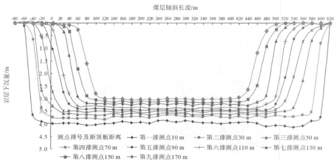
图5 工作面开采后各排测点下沉量图
