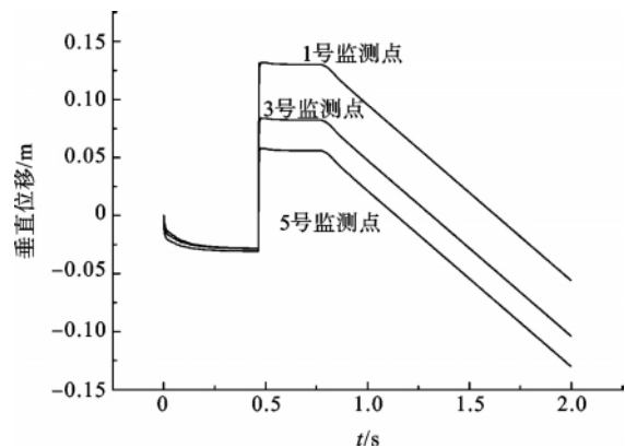
图 12 底板监测点垂直位移图(U型钢支护)
