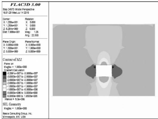
图 9 垂直应力分布云图(U型钢支护)
