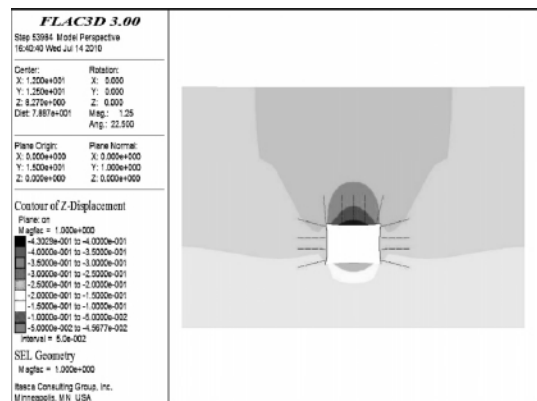
图 5 垂直位移分布云图(锚网锚杆支护)
