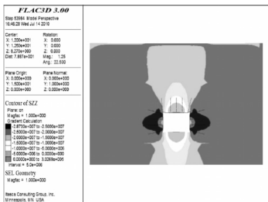
图 4 垂直应力分布云图(锚网锚杆支护)
