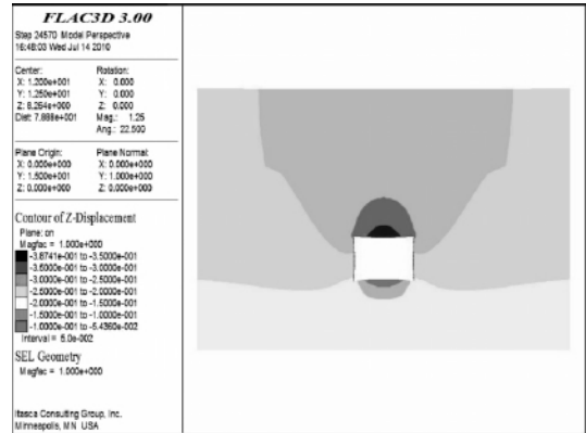
图 10 垂直位移分布云图(U型钢支护)
