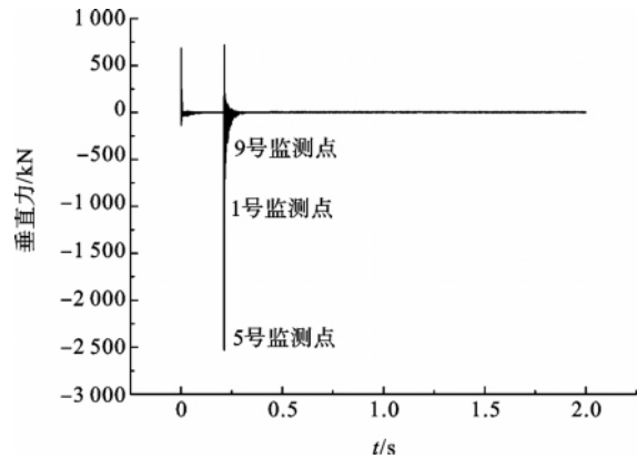
图6 顶板监测点垂直力分布图(锚网锚杆支护)
