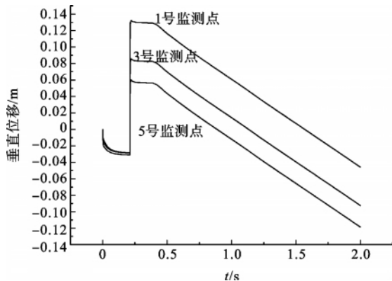
图7 底板监测点垂直位移图(锚网锚杆支护)
