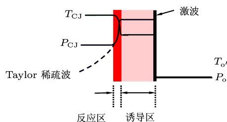
图 2 爆轰波 ZND 模型及其物理示意图
