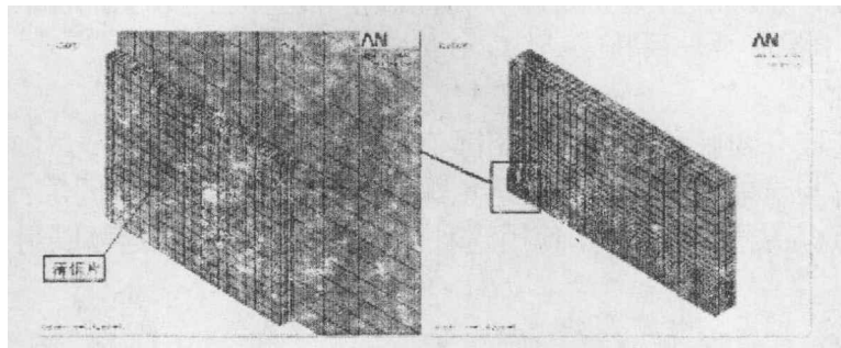
图 6 有限元计算模型
