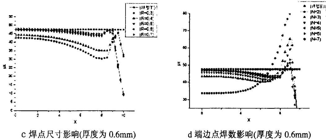
图 7. Y=0 微应变随 X 坐标的变化曲线
