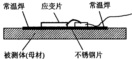
图 1 薄片应变传感器示意图
