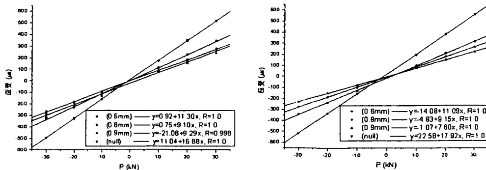
图 5 静态拉压的力—应变关系
