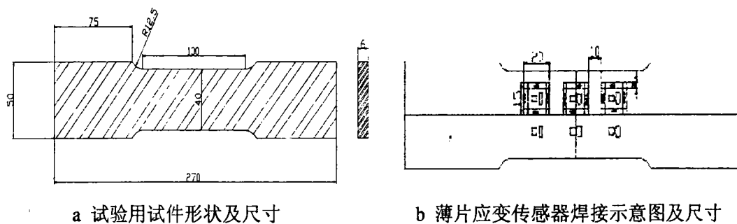
图 2 薄片应变传感器试样设计图
