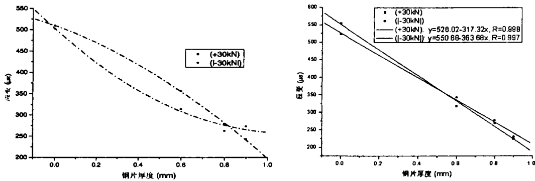
图 3 疲劳试验动态采样
