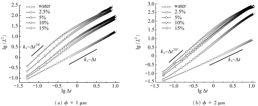
图 1 Janus 微球的 \lg \langle L^2 \rangle \sim \lg \Delta t 曲线
