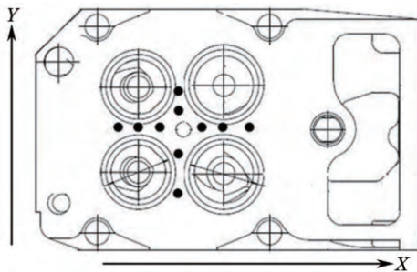
图1 气缸盖火力面测点分布示意图
