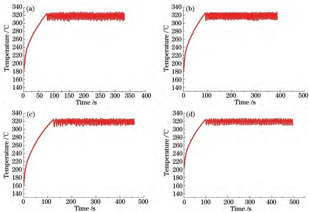
图8 温度控制的通气冷却高周热负荷试验。(a) 3000 W; (b) 2800 W; (c) 2600 W; (d) 2500 W
