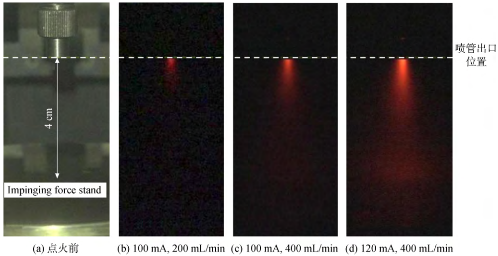
图 2 不同条件下推力器喷管和羽流照片
