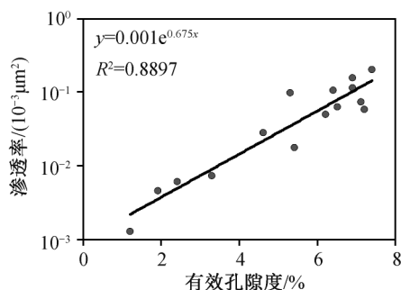
图5 盐池地区长8储层样品渗透率与有效孔隙度的关系
