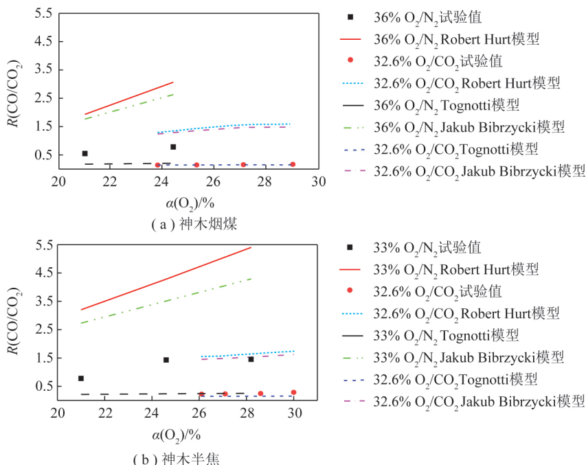
图 2 不同预热气氛下预热气体组分 CO/CO 2 试验结果及模型值
