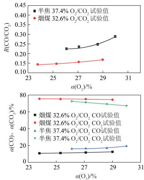
图4 不同燃料的试验结果对比
