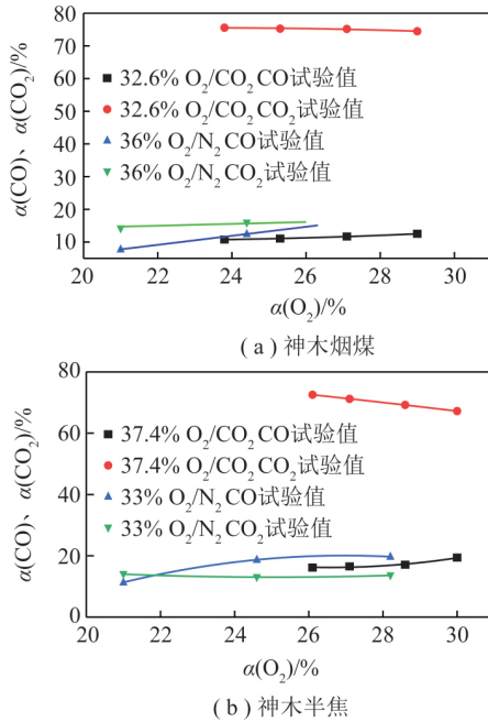
图3 不同预热气氛下试验结果
