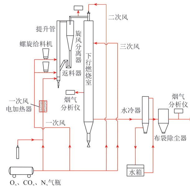
图 1 试验系统工艺流程 [13]
