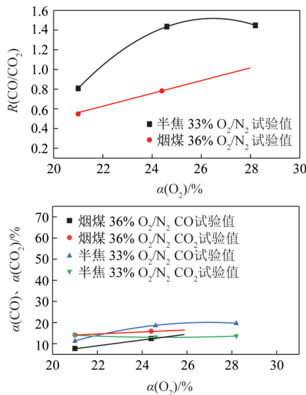
图4 不同燃料的试验结果对比
