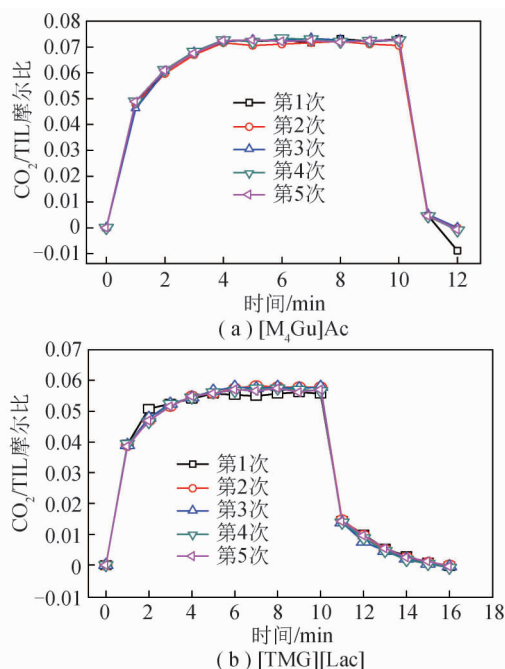
图3 离子液体在 70 °C 下重复吸收/解吸收 CO_2 特性
