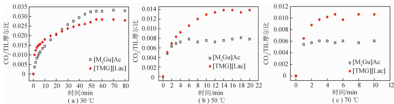
图 4 常压条件下 [M 4 Gu]Ac 和 [TMG][Lac] 对水泥窑窑尾烟气中 CO 2 吸收特性
