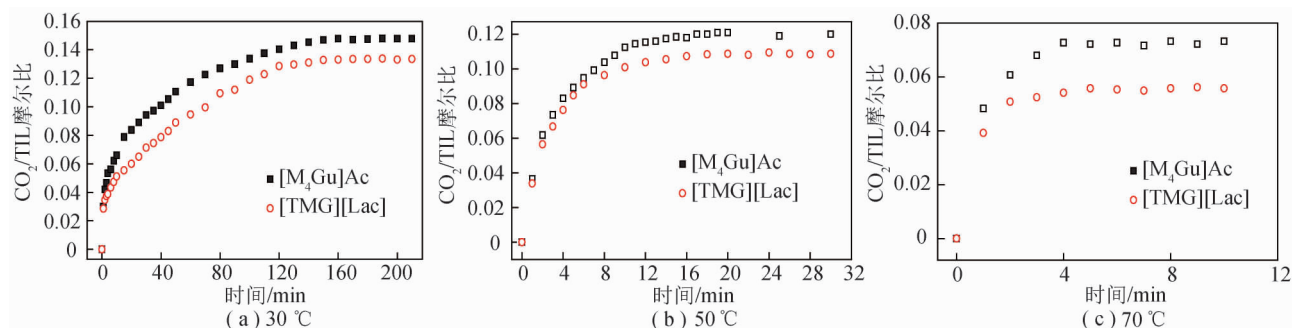
图2 常压条件下 [M_4Gu]Ac 和 [TMG][Lac] 对 CO_2 吸收特性
