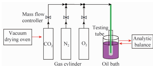
图1 离子液体吸收CO 2 试验系统
